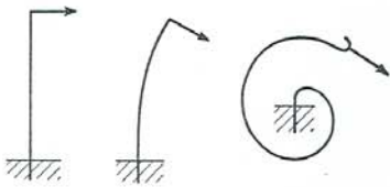
Fig. 14. — Le ressort spiral est un ressort de flexion
