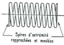
Fig. 19. Ressort à compression
