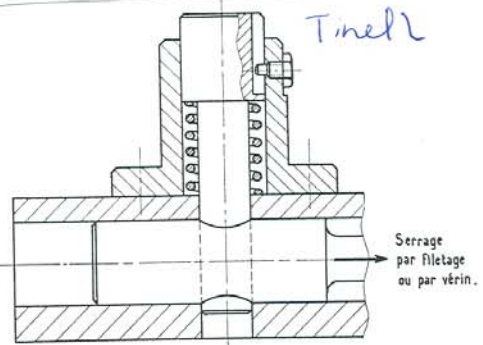
Fig. 23. Butée à ressort, pour montage d'usage.
