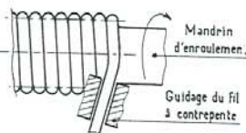
Fig. 22. Le précédent, en fabrication.
