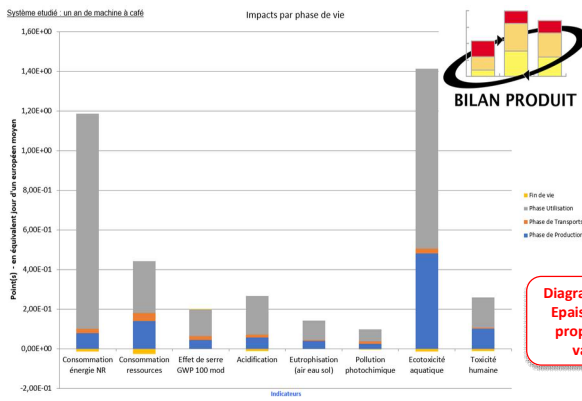
[ADEME (2011) Exemple de la machine à café du logiciel Bilan produit]
