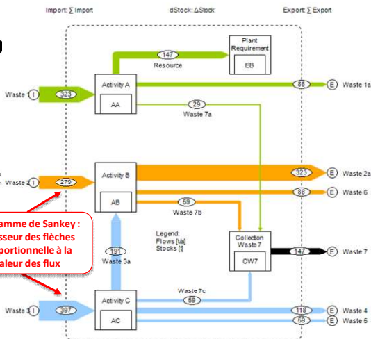
[Fichier « Exemple from Austrian Standard S2096, 2006 » fourni avec le logiciel STAN 2.7.101]
