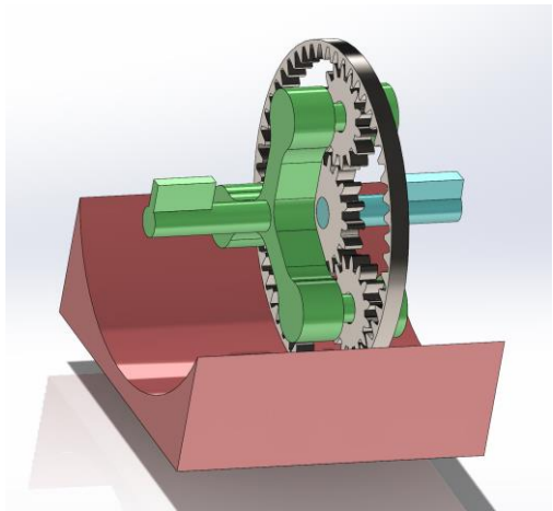
Train épicycloïdal
