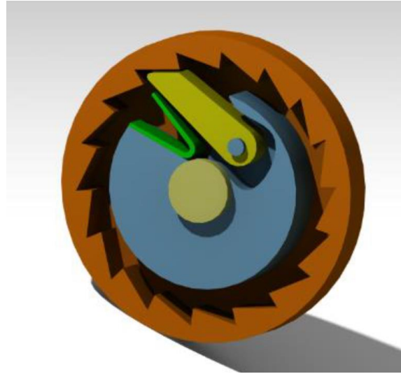
Roue libre
