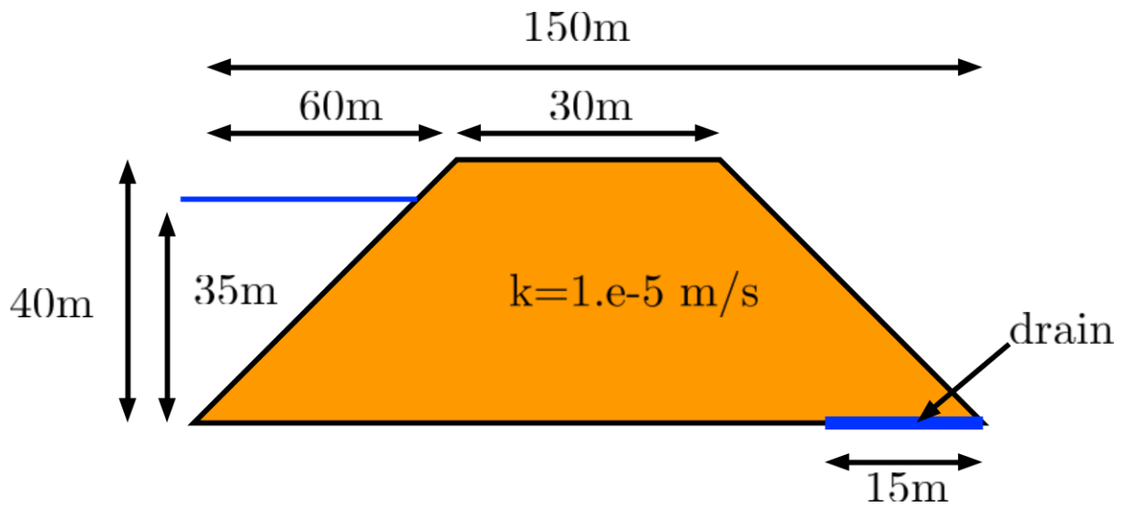
Figure 1 : données géométriques et conditions limites
