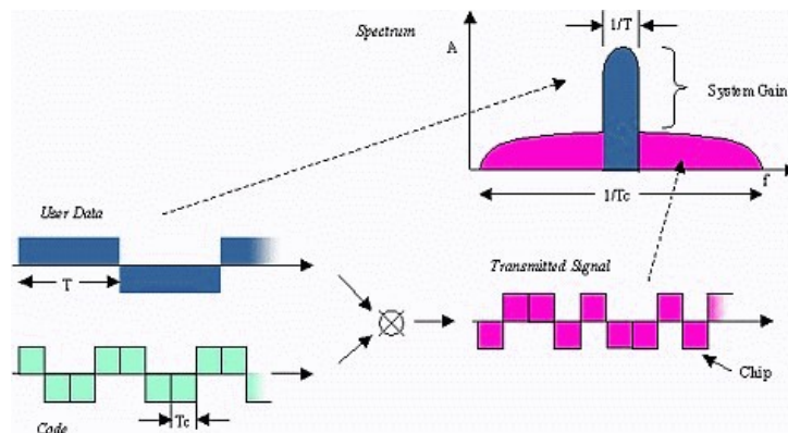
— DSSS —
