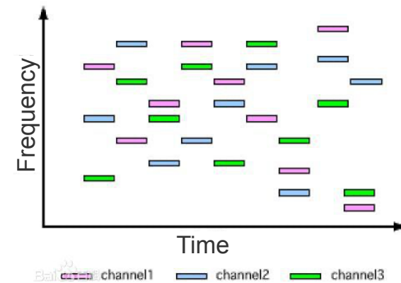
— FHSS —
